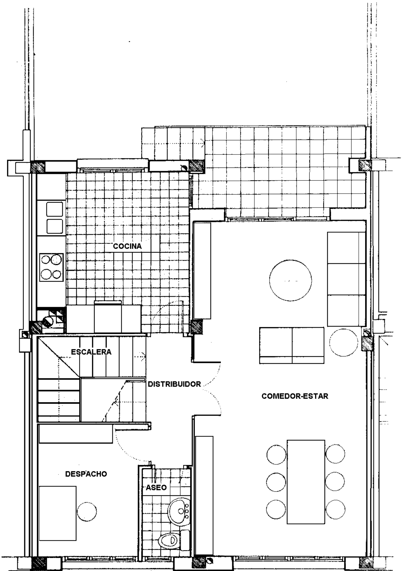
PLANTA PRIMERA (superficies aproximadas)
