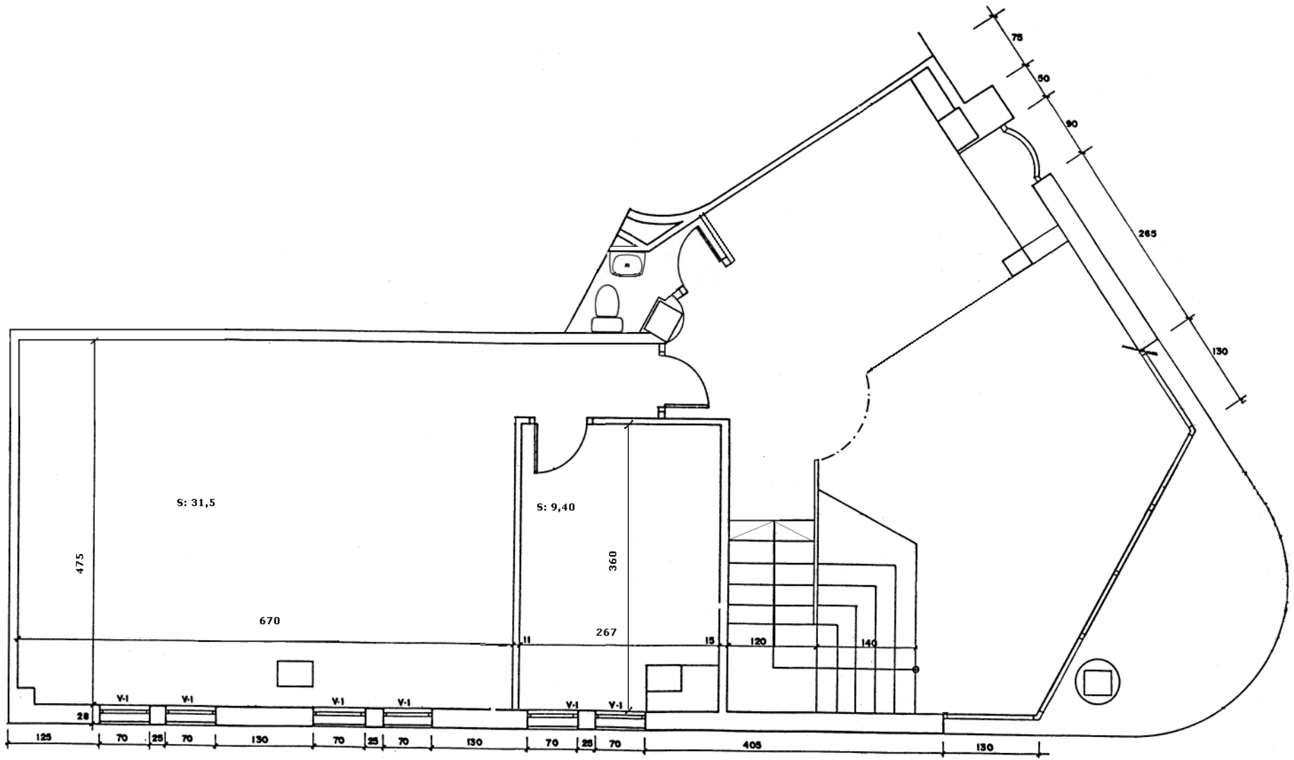
PLANTA ALTILLO
